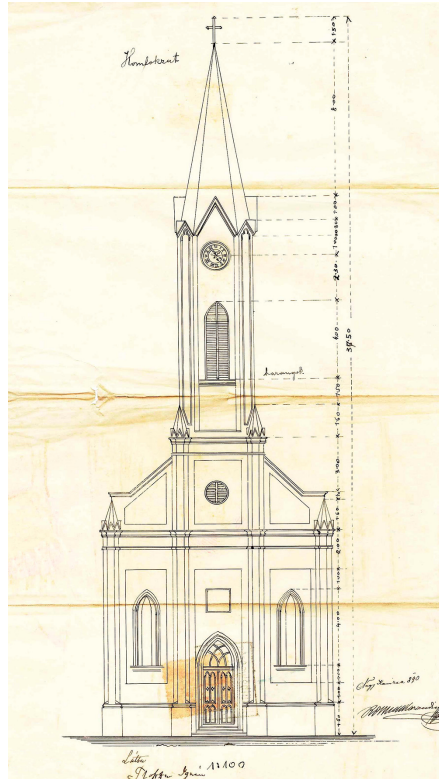
Az 1891-ben felavatott evangélikus templom terve (Csengery út 37.)
