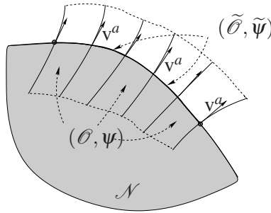
12.1. ábra. Az (\mathcal{O}, \psi) térkép előállítását a v^a vektormező segítségével.
