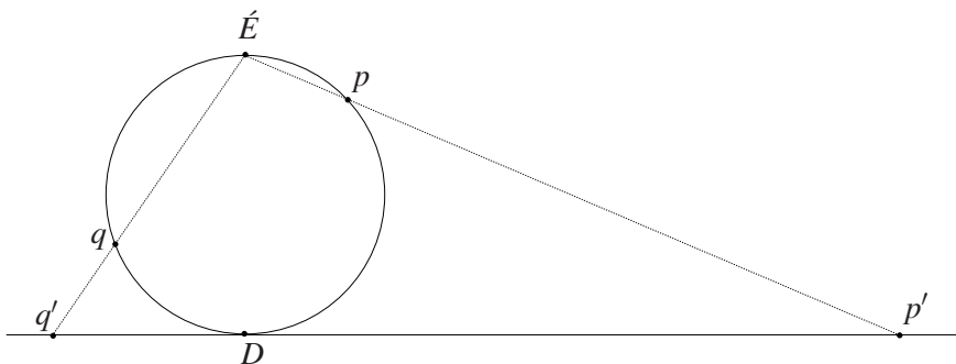
2.2. ábra. Az északi pólusból elvégzett \psi_{\acute{E}} sztereografikus projekció hatásának megjelenítése.
