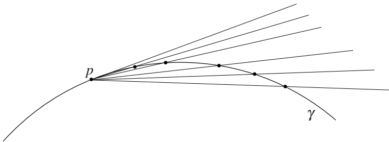
2.4. ábra. A \gamma görbe p pontjából indított szelőinek határ-félegyeneseként előálló érintő – a választott parametrizációnak megfelelően irányított – félegyeneset határoz meg.
