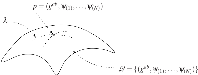
14.1. ábra. Az illusztrációnak szánt felület nemcsak a \mathcal{Q} konfigurációs teret, de a hatásnak, mint funkcionálnak egy megvalósuló fizikai állapot közelében való lehetséges viselkedését is jelzi.
