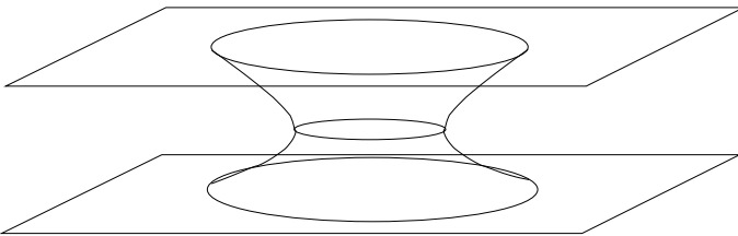
18.5. ábra. A Schwarzschild-téridő maximális analitikus kiterjesztésében a \frac{T}{X} = \text{állandó} hiperfelületek topológiájának illusztrációja. A minimális sugarú kör az r = 2M sugarú bifurkációs gömbfelületet jeleníti meg.
