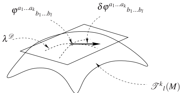
14.2. ábra. Tenzormezők egyparaméteres variációinak illusztrációja.
