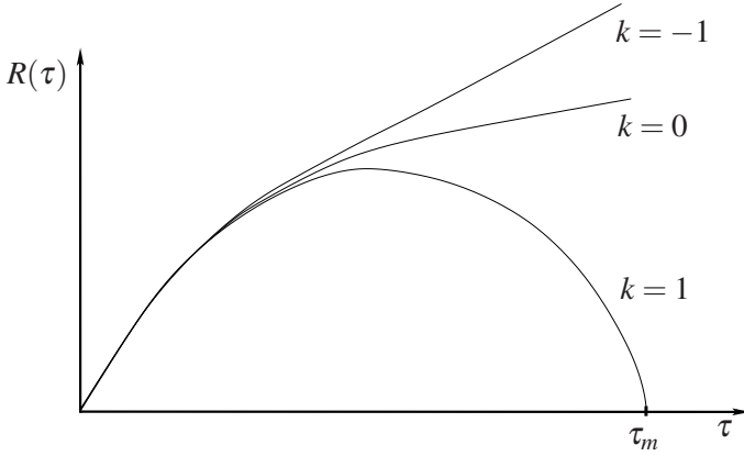
17.8. ábra. A Friedmann-univerzum R(\tau) skálafaktorának kvalitatív viselkedése az állandó görbületű terekre vonatkozó három lehetséges állapot figyelembevételével.
